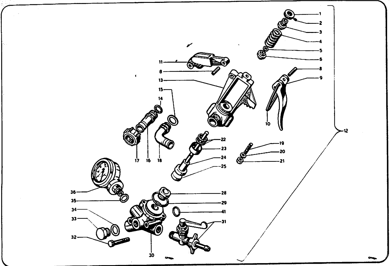
NOMENCLATURA RICAMBI POMPA 45S TAV. 3
